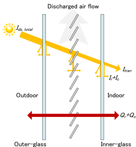
Gambar 3. Ilustrasi Transfer pada Fasad Selubung Ganda
