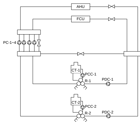
Gambar 8. Diagram Sistem Pengkondisian Udara
