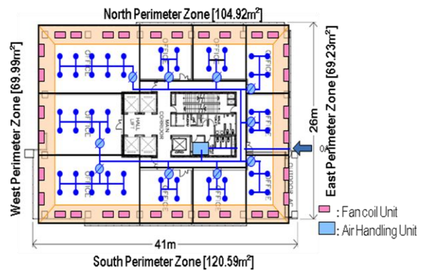
Gambar 7. Zoning AHU dan FCU
