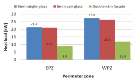
Gambar 5. Beban Panas Puncak pada Zona Perimeter.
