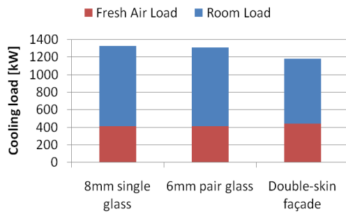
Gambar 6. Beban Pendingin dan tip Selubung.
