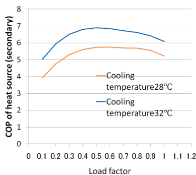
Gambar 9. Load Characteristic dari Heat Source
