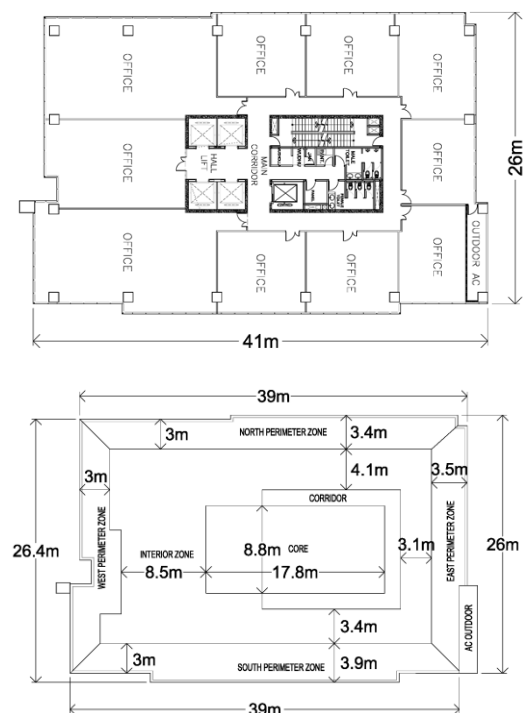
Gambar 2. Tipkal Lantai dan Zona Perimeter
