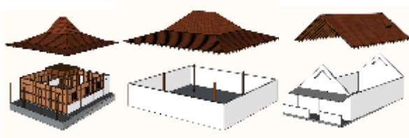
Gambar 6a (kiri). Rancangan atap Joglo . Gambar 6b (tengah). Rancangan atap Limasan. Gambar 6c (kanan). Rancangan atap dapur.
