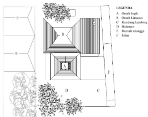
Gambar 4. Siteplan objek penelitian.
