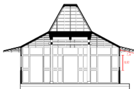
Gambar 10. Lebar tritisn bangunan.
